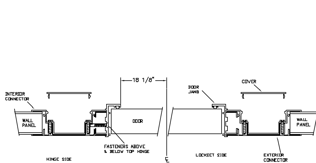
3068 DOOR FRAME
