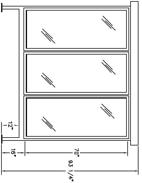
ELEVATION A
