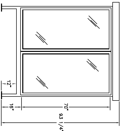
ELEVATION A
