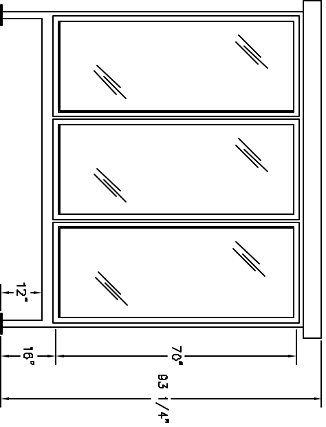
ELEVATION A
