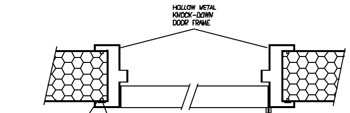
DOOR SECTION
