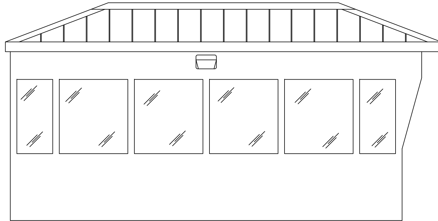
ELEVATION A
