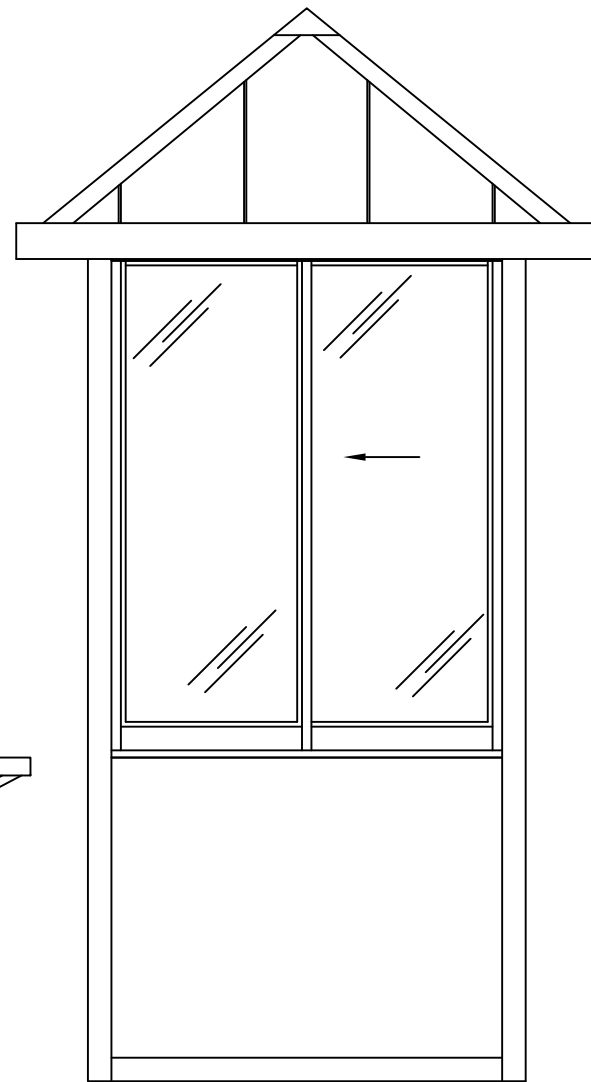
ELEVATION B
