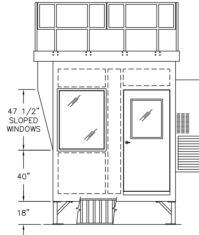
ELEVATION B
