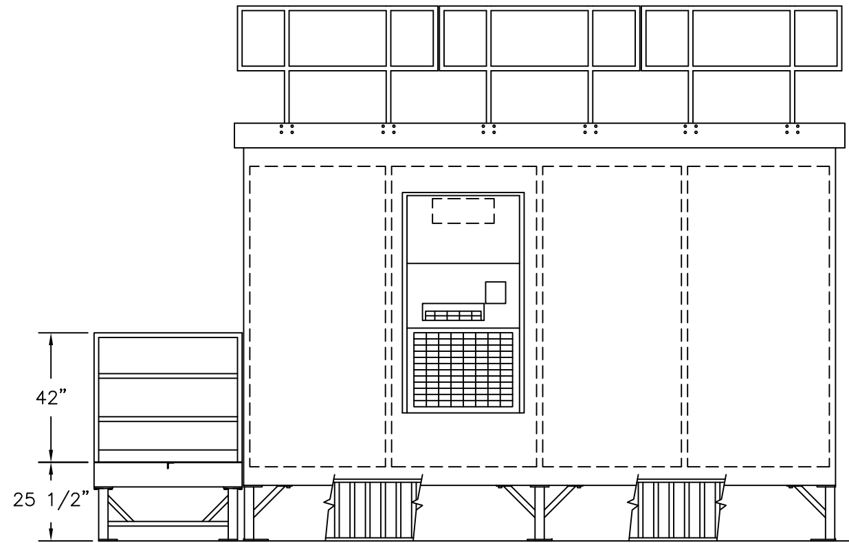
ELEVATION A
