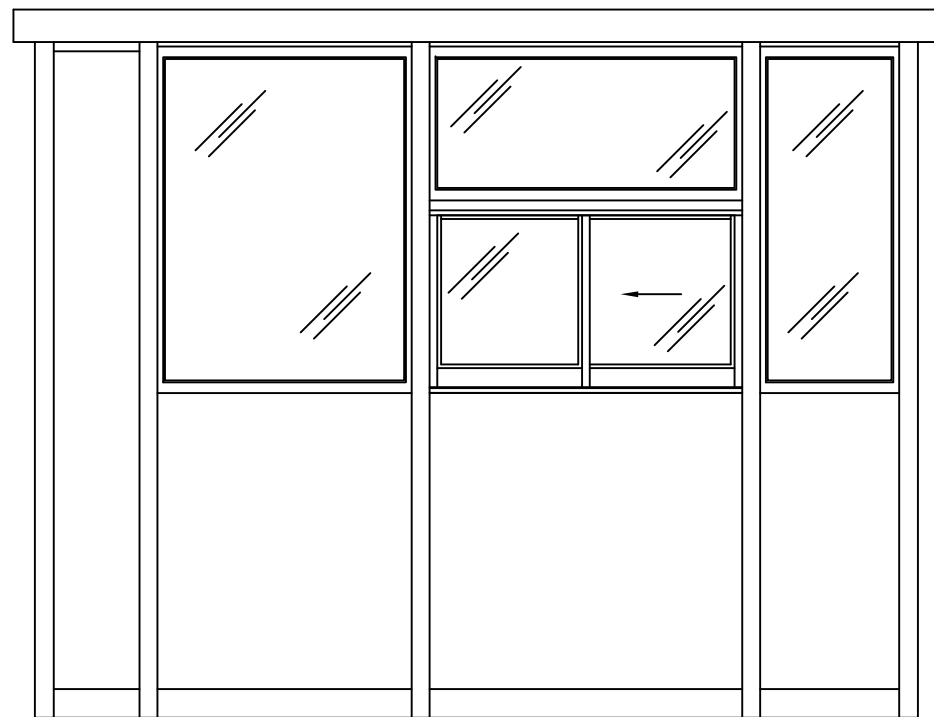
ELEVATION A
