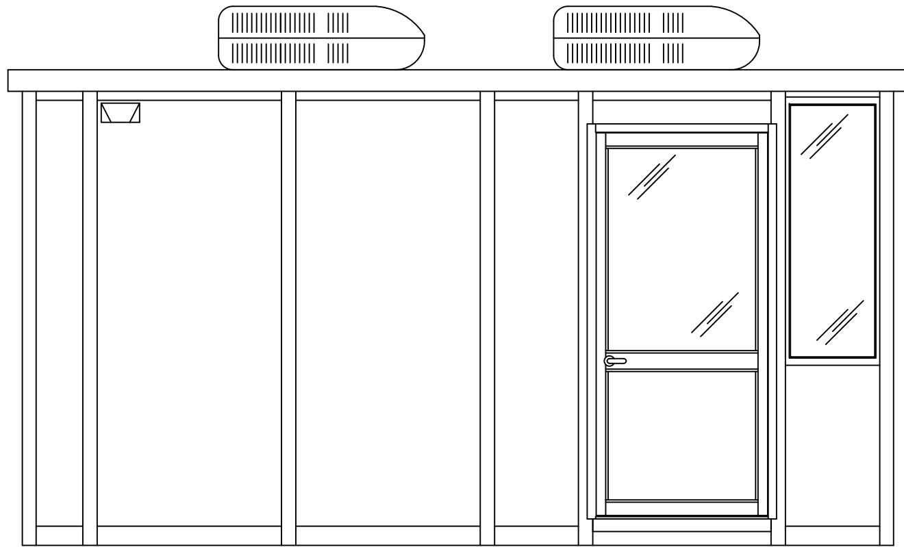
ELEVATION A
