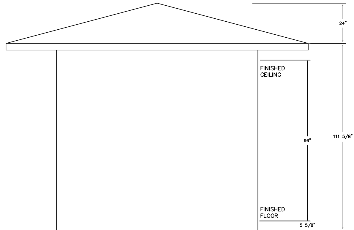
ELEVATION B
