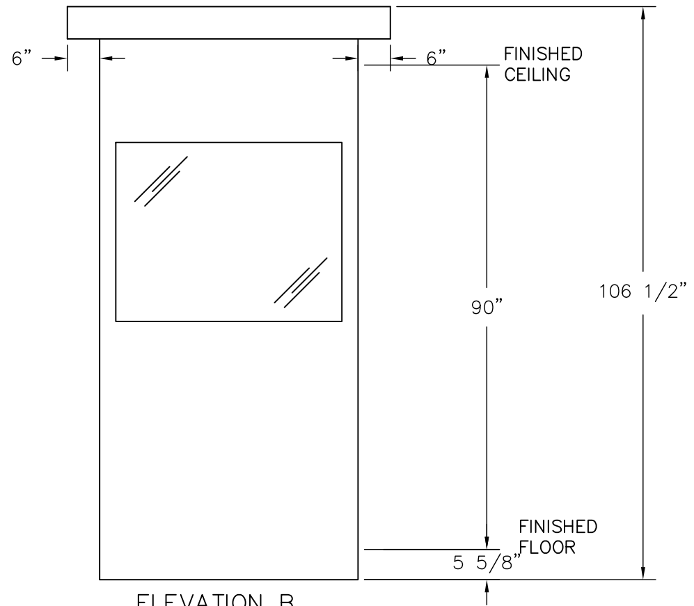
ELEVATION B
