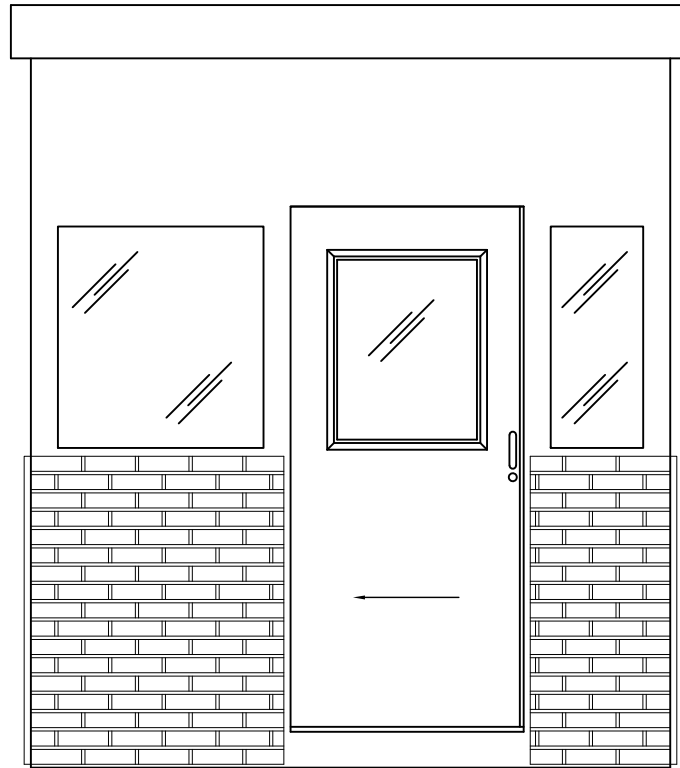
ELEVATION A
