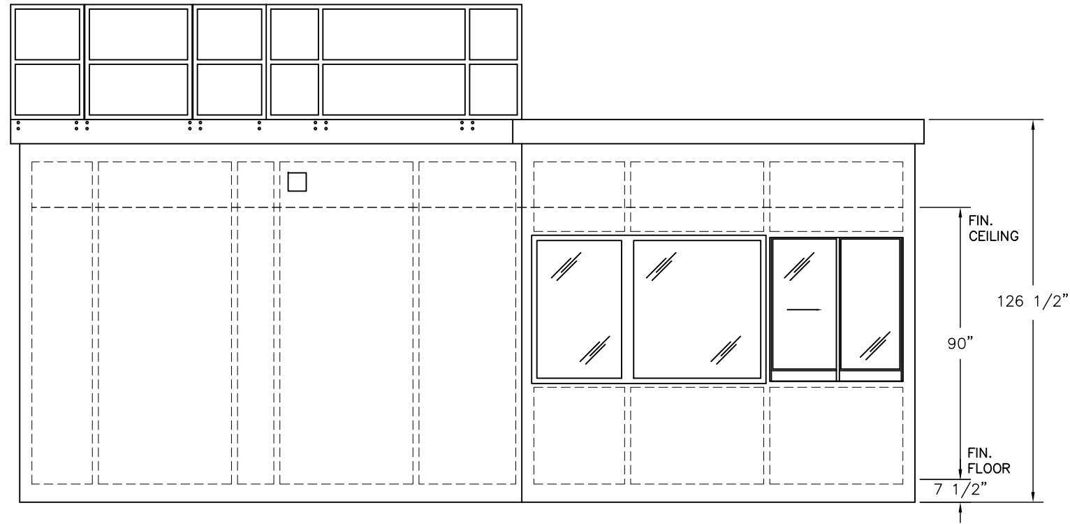
ELEVATION A
