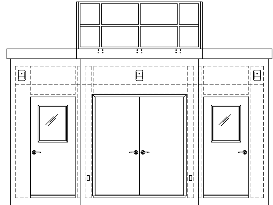
ELEVATION B
