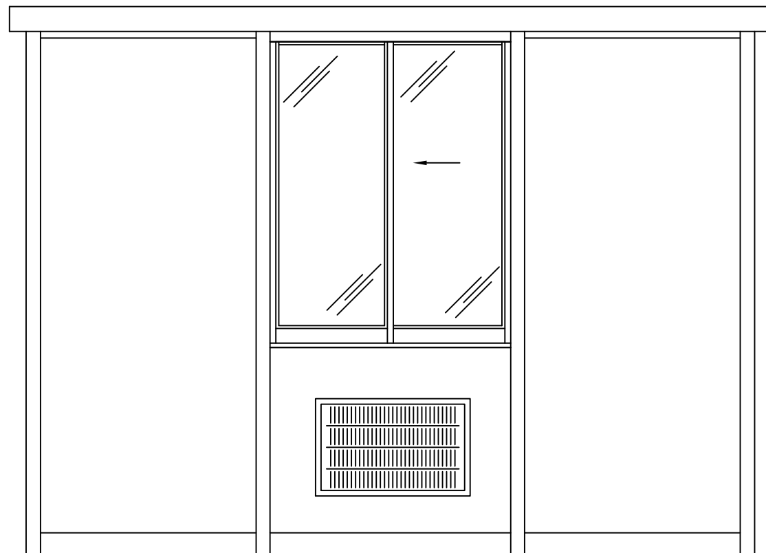
ELEVATION A
