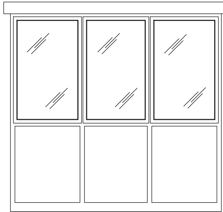
ELEVATION B
