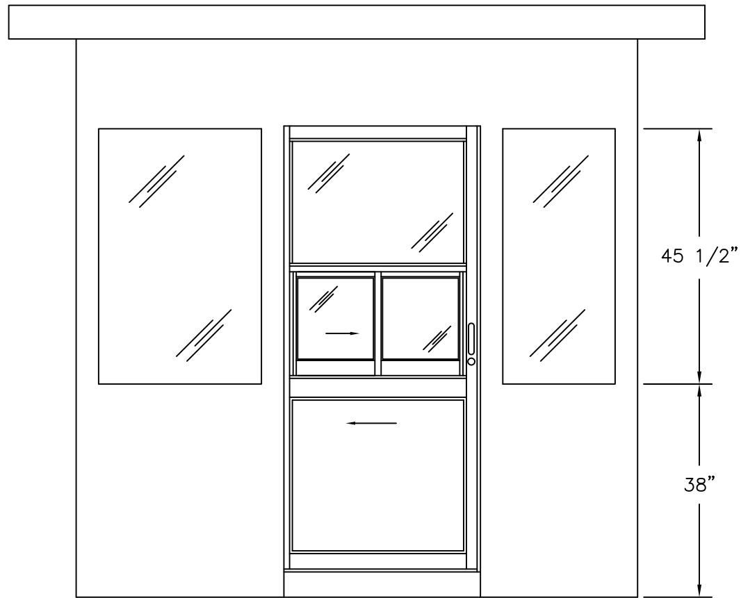
ELEVATION A
