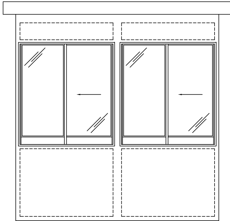
ELEVATION A
