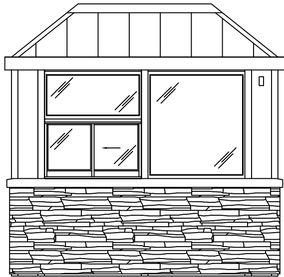
ELEVATION A
