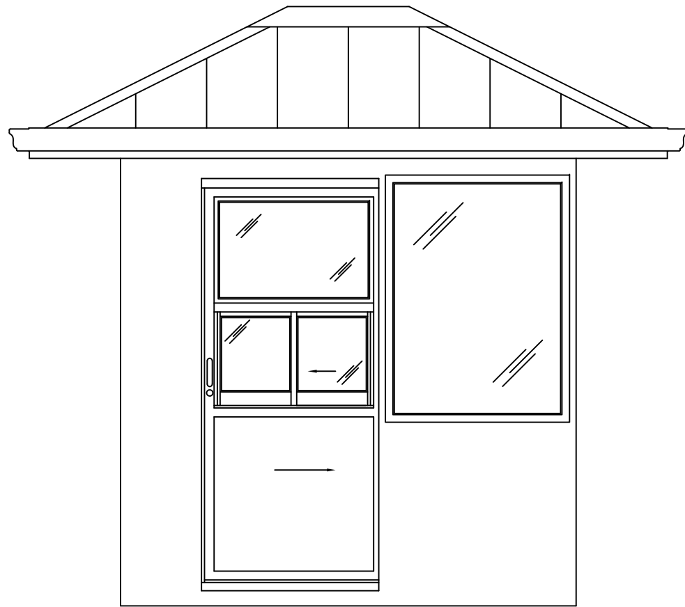
ELEVATION A
