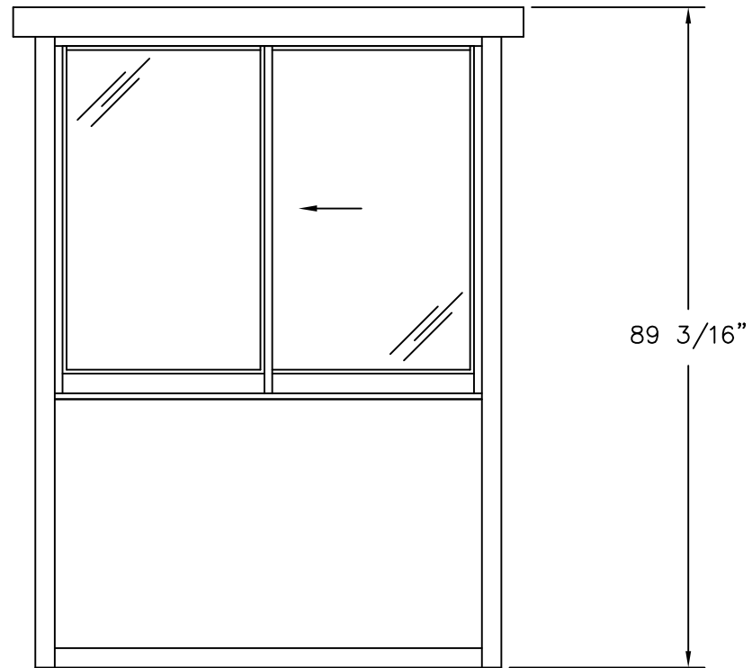
ELEVATION B
