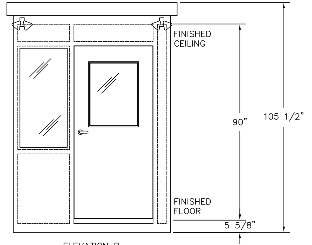
ELEVATION B
