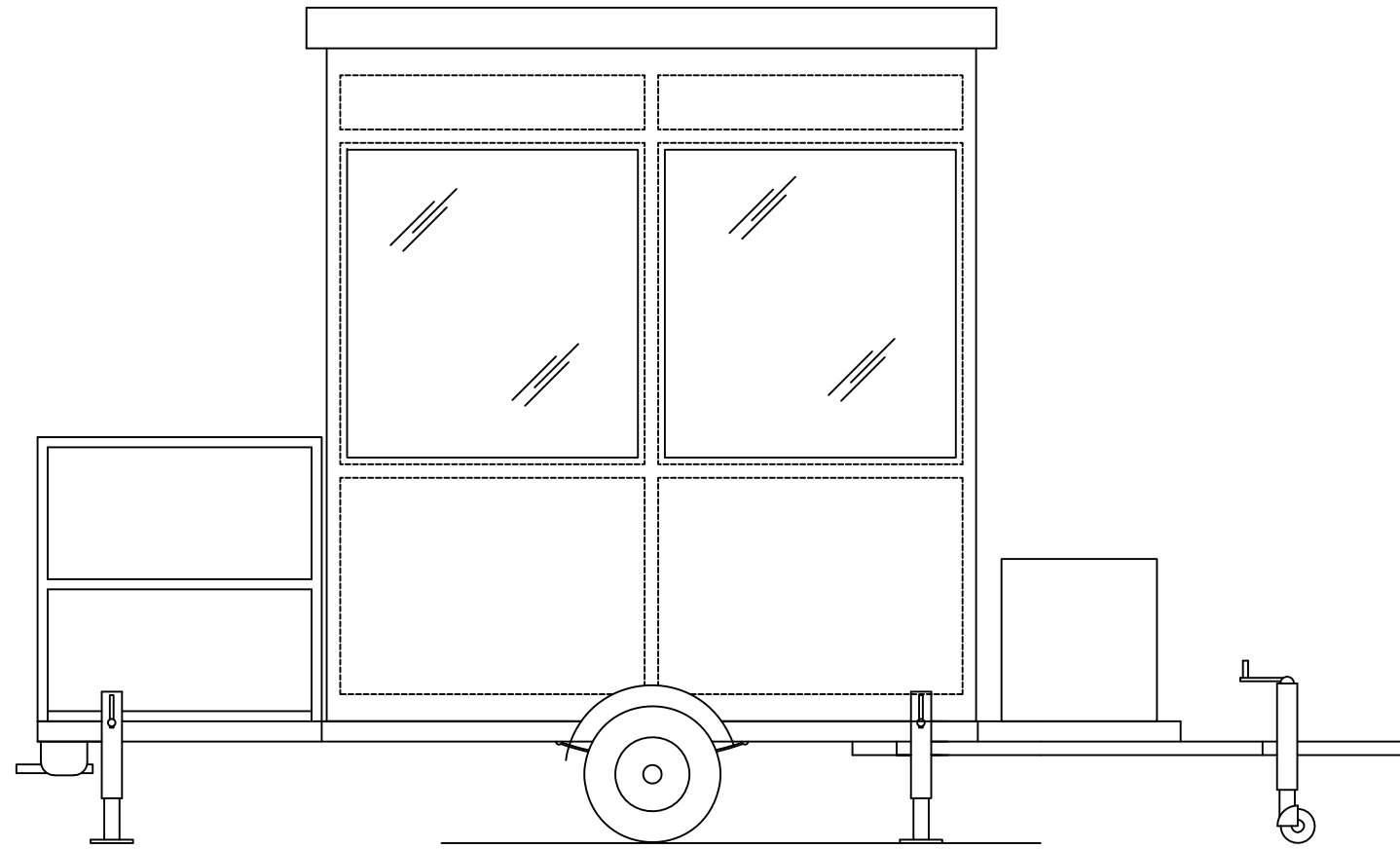
ELEVATION A
