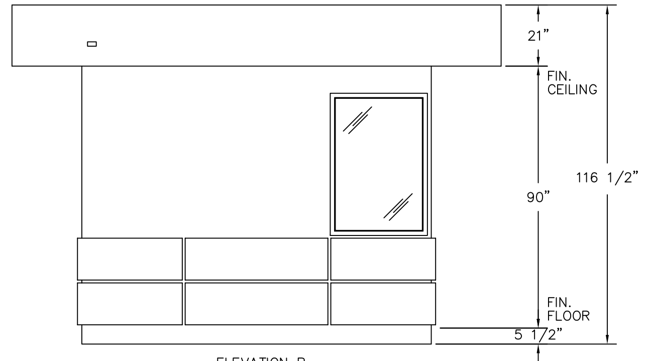
ELEVATION B
