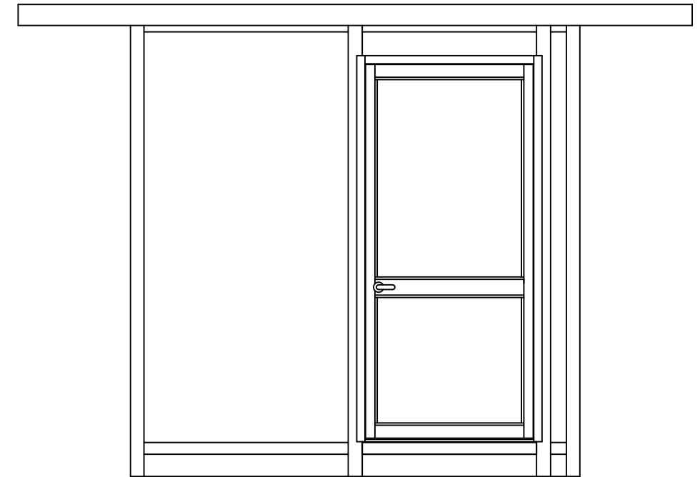
ELEVATION B
