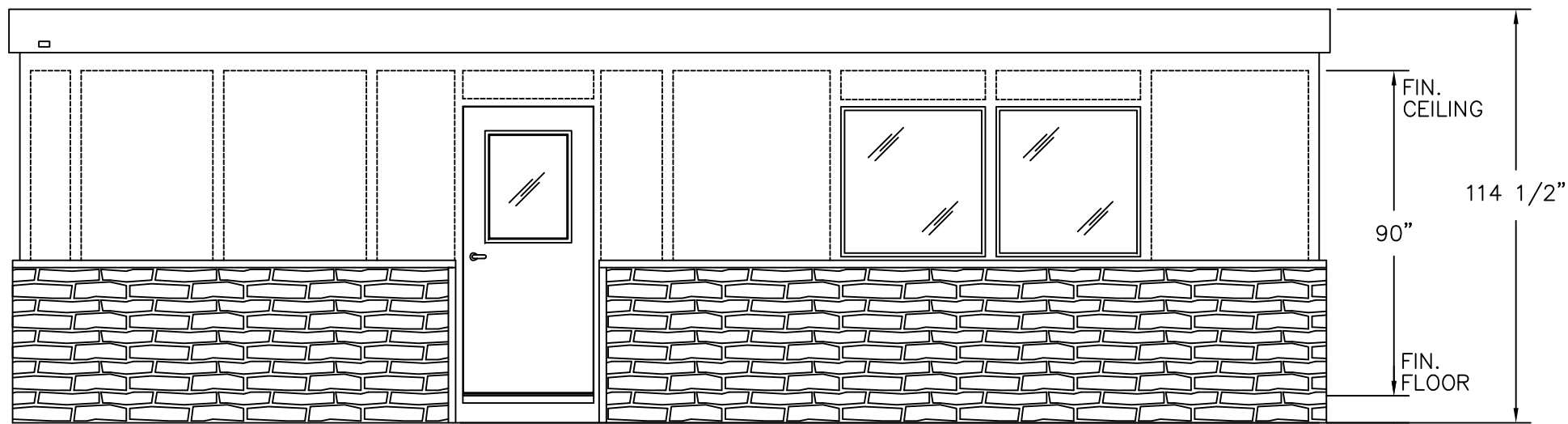
ELEVATION A
