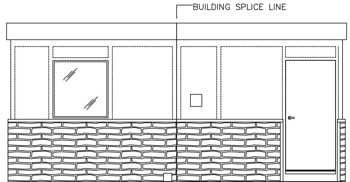
ELEVATION B
