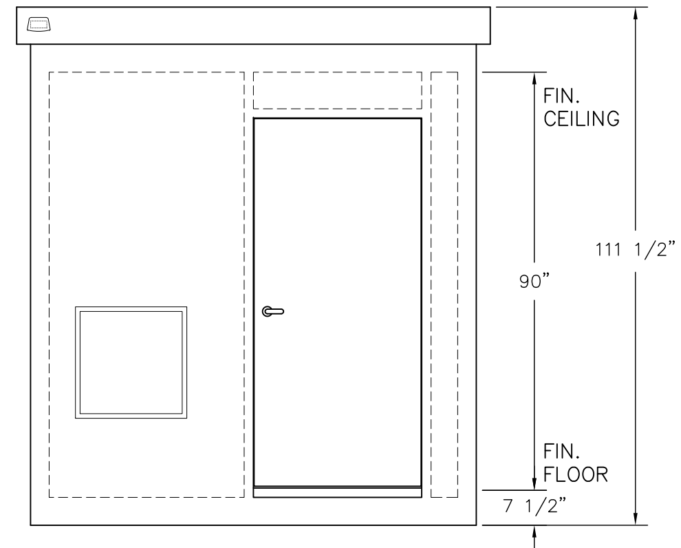
ELEVATION B
