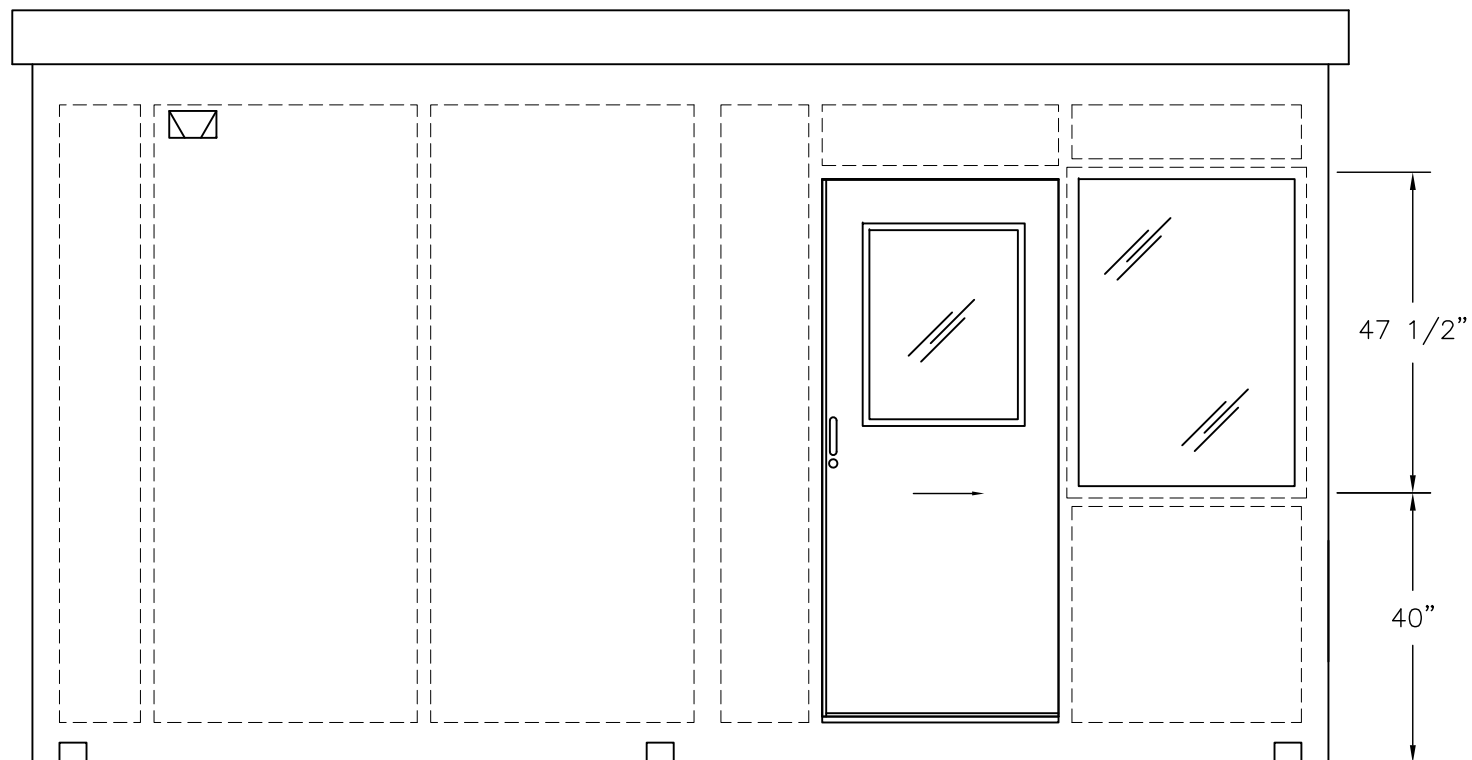
ELEVATION A
