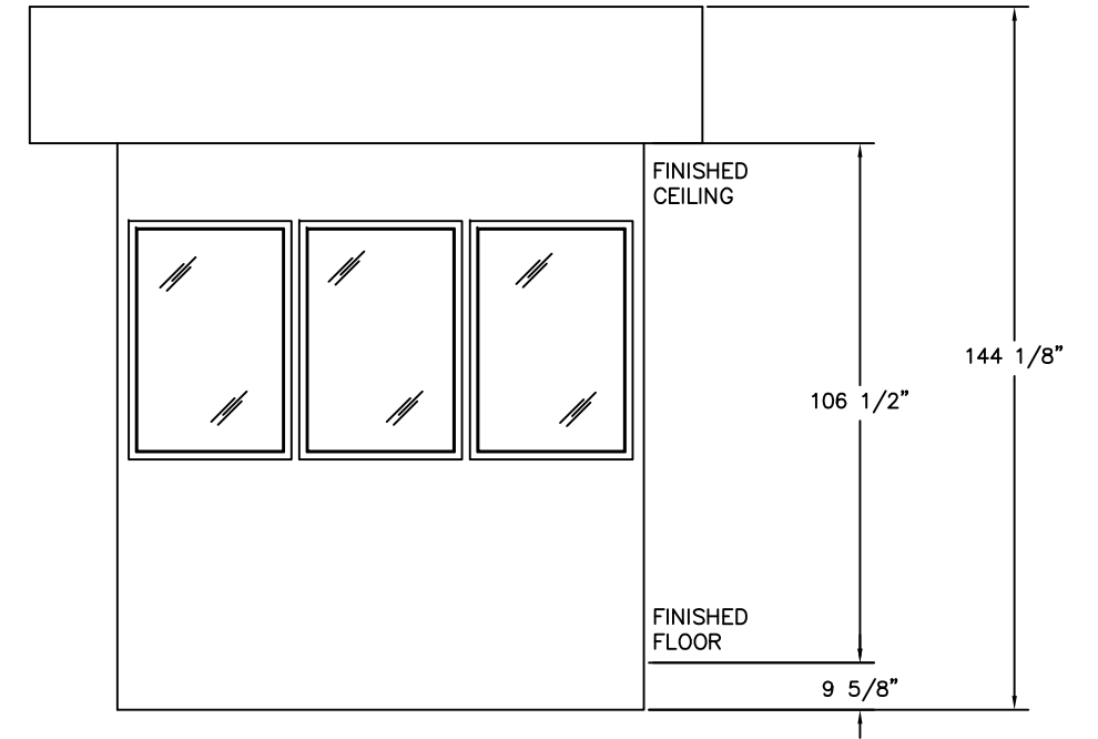
ELEVATION B
