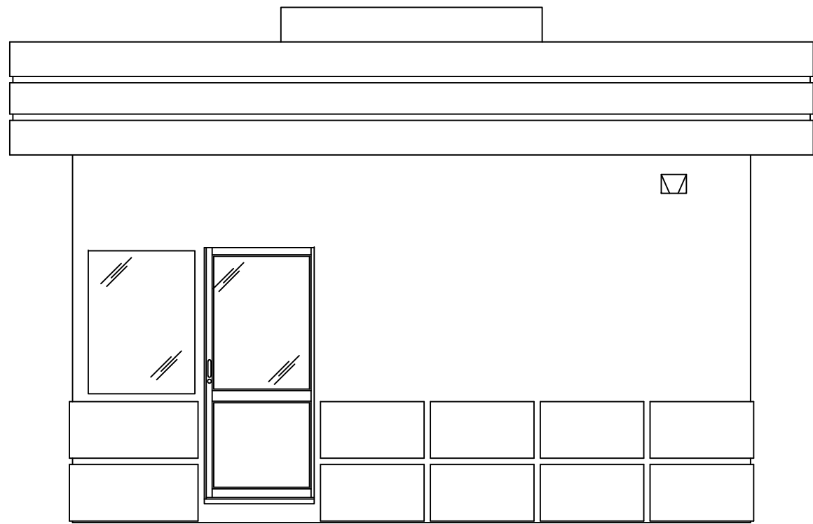
ELEVATION A
